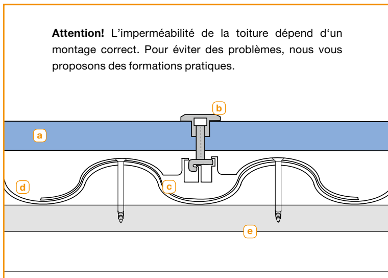
Vue latérale
